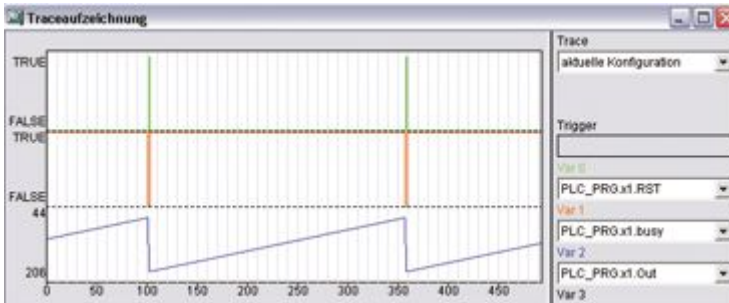
Timing Diagramm für Sägezahngenerator:
