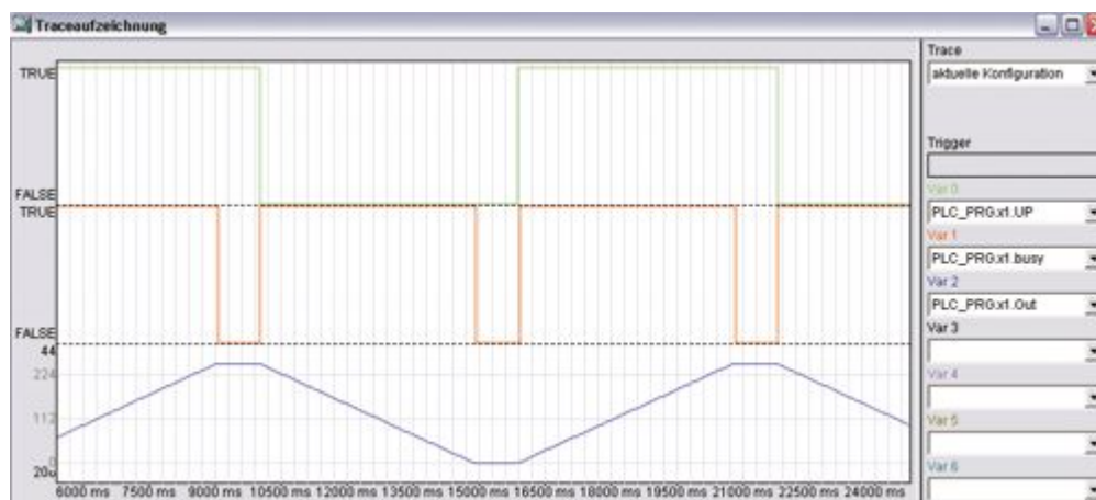
Timing Diagramm für Up / Down Rampe:
